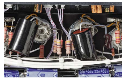
W okolicach lamp dominują połączenia punkt-punkt, pozostałe układy zmontowano na płytkach drukowanych.
